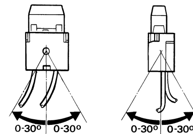
рис. 26: Держатель предохранителя, положение установки
