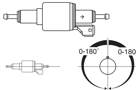
рис. 16: Дозирующий насос DP 30.2/30.3 Положение установки
