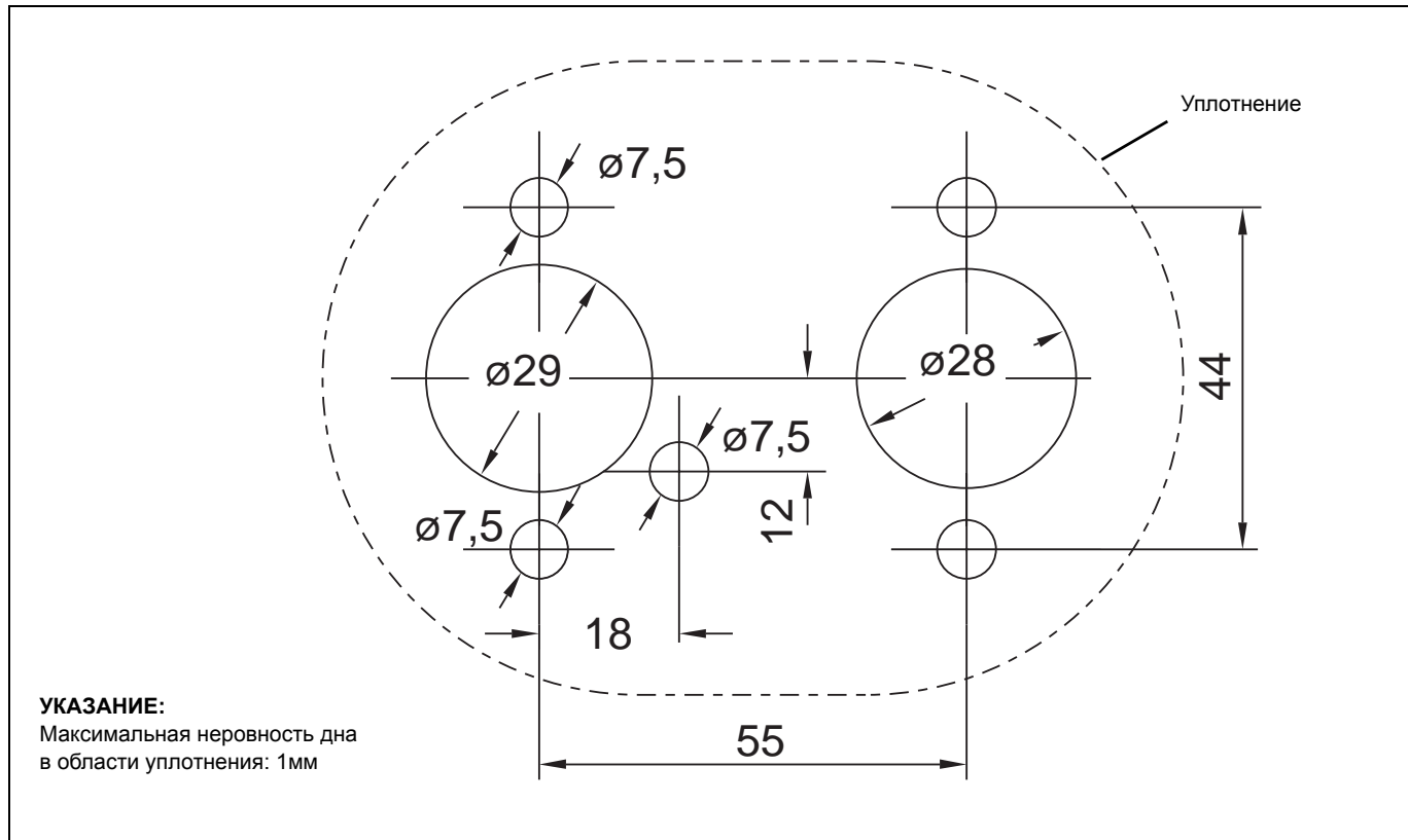
рис. 35: Шаблон отверстий
