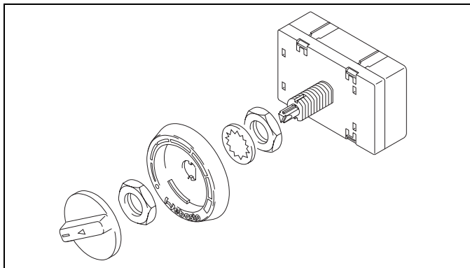
рис. 27: Орган управления
